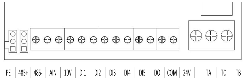
图 3：DS120 端子示意图
