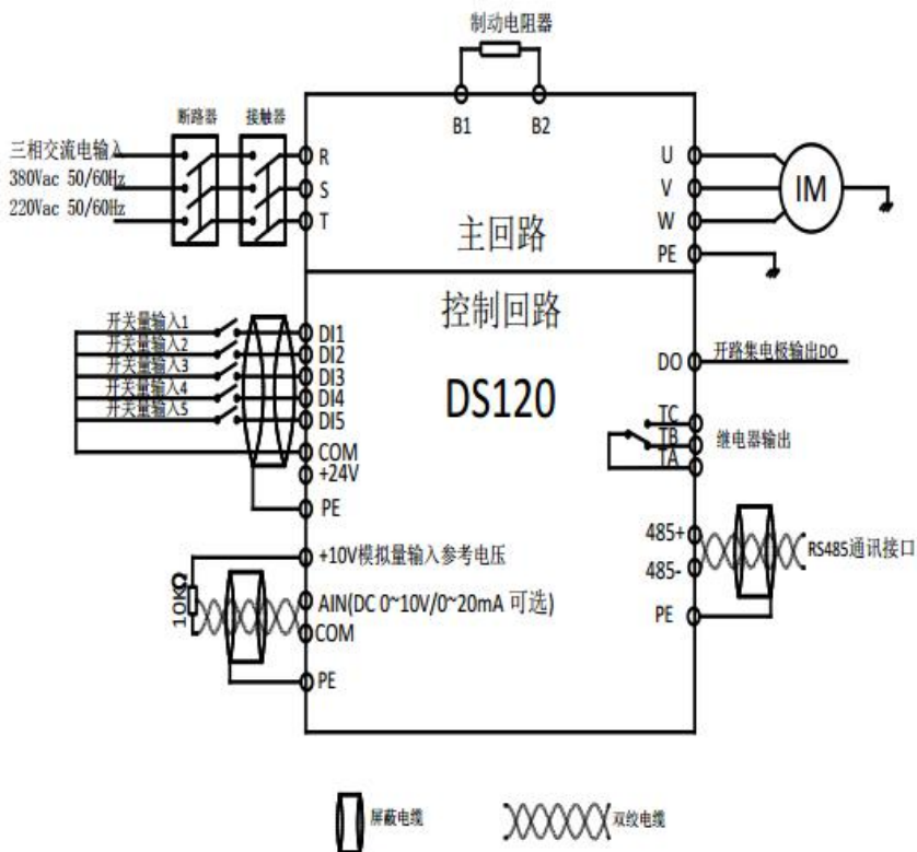
图 6：DS120 变频器主回路接线端子图
