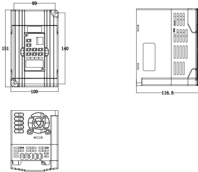
图 2：DS120 外形尺寸图
